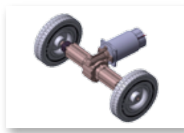
Motodifferenziale
